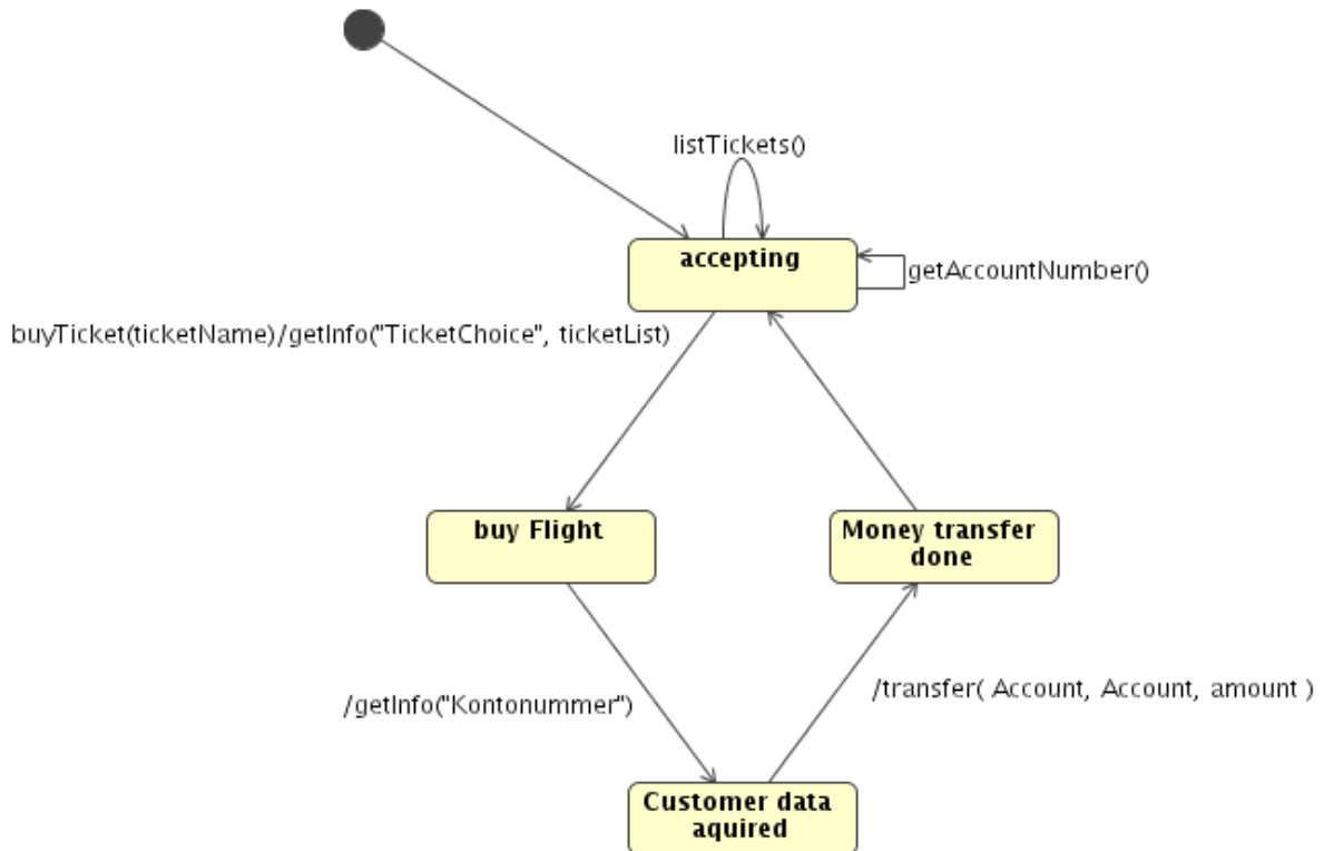
Рис. 10. Діаграма станів компонента «Авіакомпанія» (Airline).
